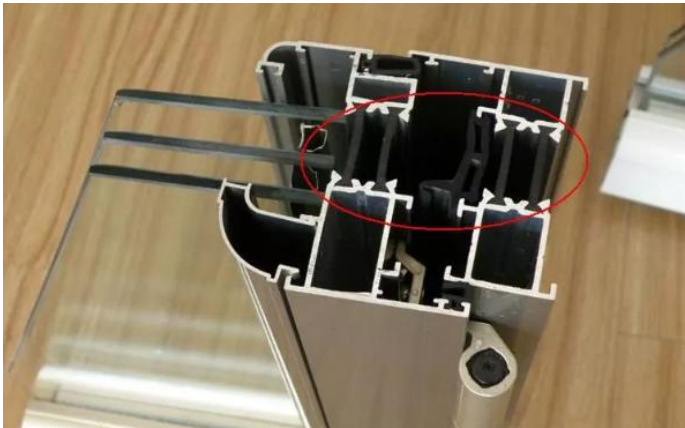
▲隔热条
